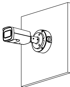
接線盒安裝
