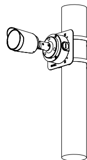
立桿安裝
