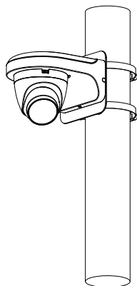
立柱安裝(垂直)
